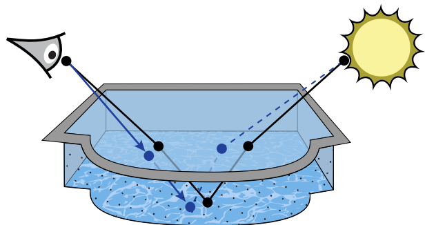
(d) Manifold perturbation
